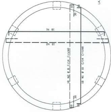
ARMACAD DO FUNDO DO RESERV. Esc.1:25 Cobrimento = 2cm
