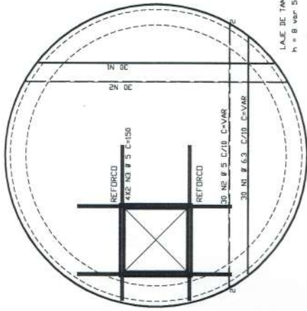
ARMACAD DA TAMPA Esc.1:25 Cobrimento = 1 cm
