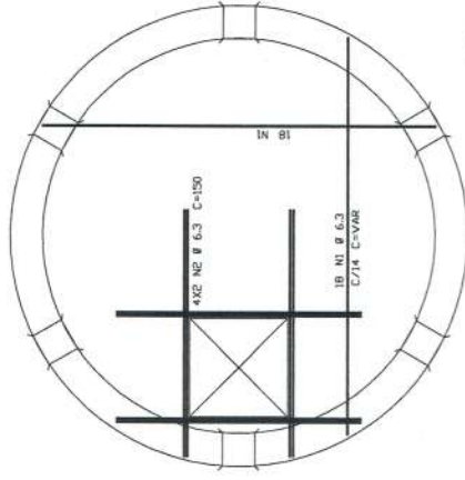
PLANTAS - NIVEIS 358 E 696 Esc.1:25 Cobrimento = 1 cm
