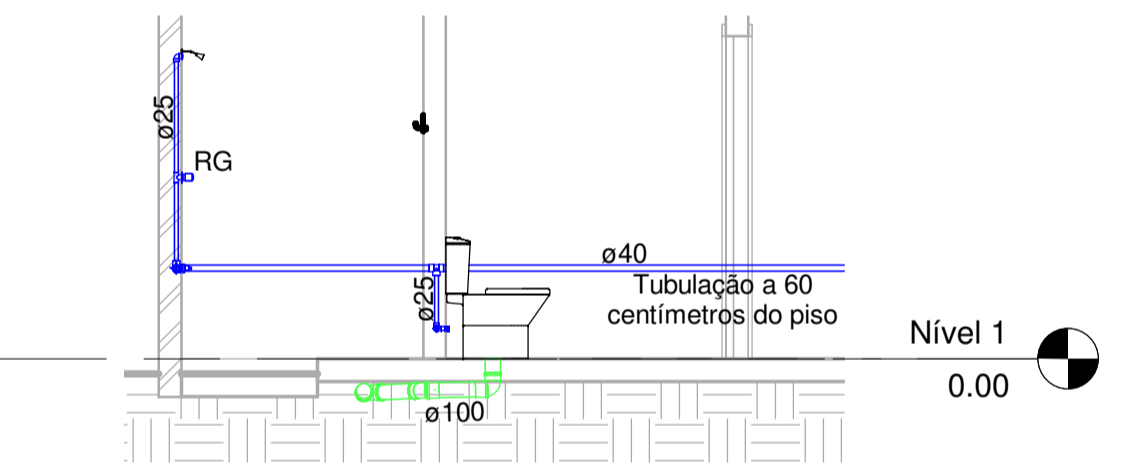
4 Detalhe Banheiro 1 : 50
