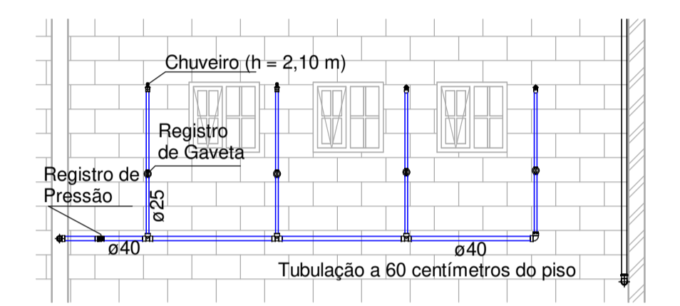
3 Detalhamento Chuveiro 1 : 50
