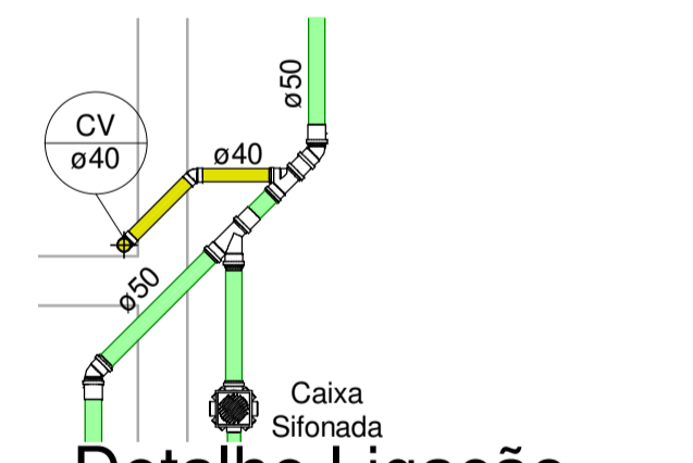
5 Detalhe Ligação Ventilação-Esgoto 1 : 25
