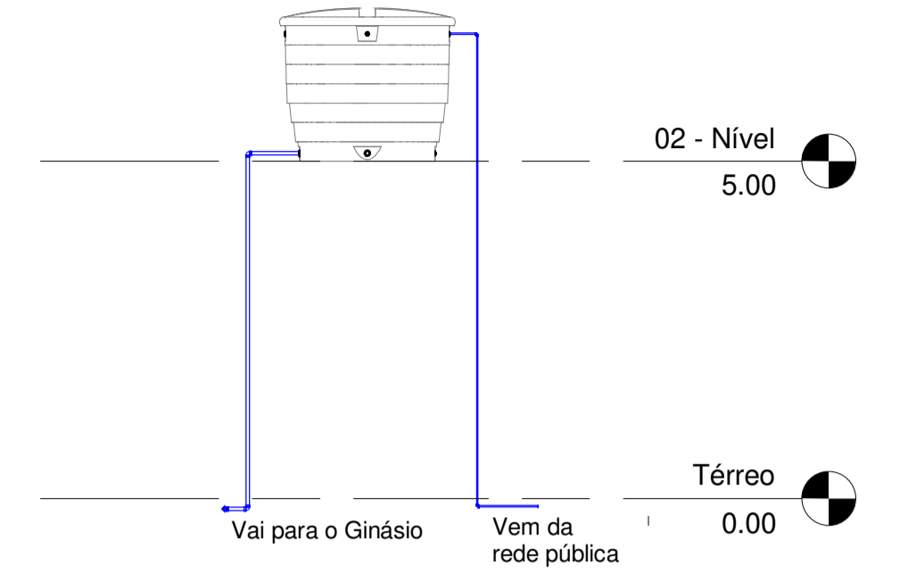
2 Detalhamento Reservatório 1 : 100
