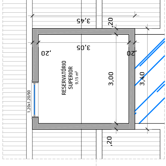
— ARQ RESERVATÓRIO SUPERIOR ESCALA - 1/75
